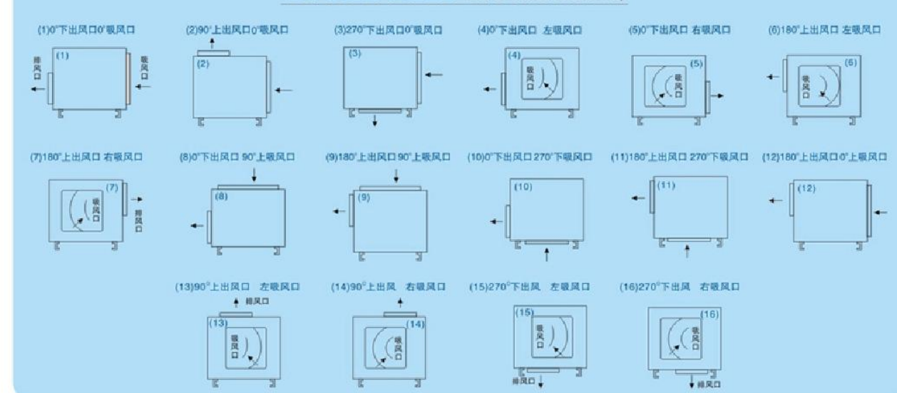
柜式风机进风口位置图 Inlet &amp; Outlet Location Map
